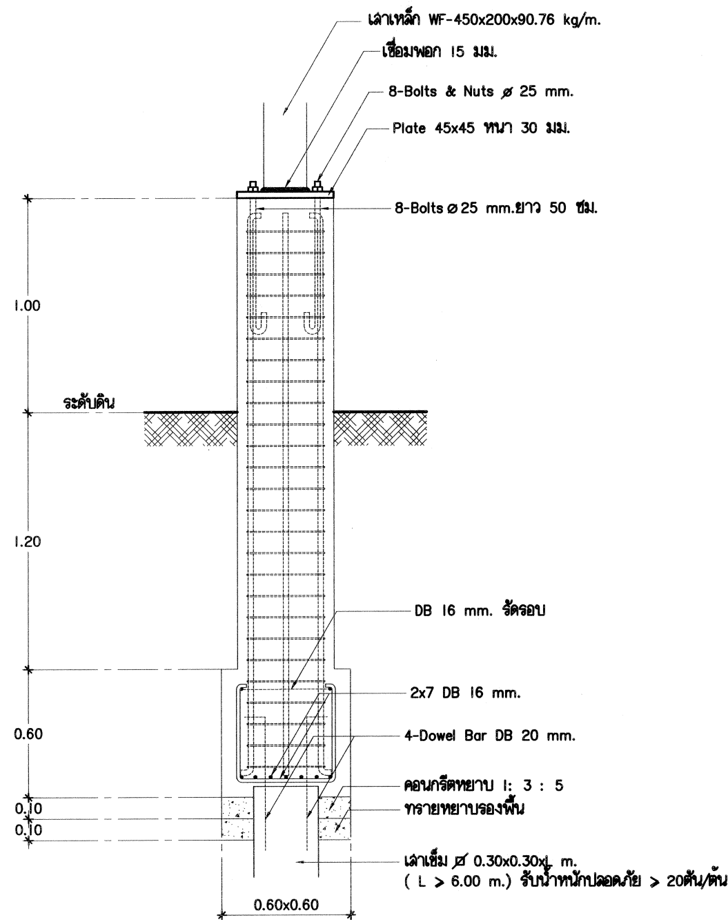
ขยายฐานราก F-1
