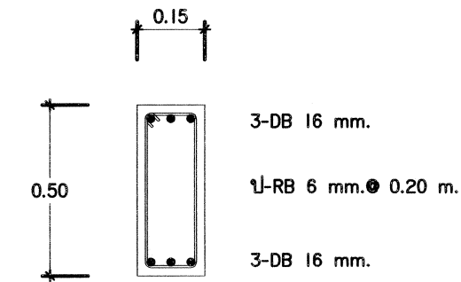
ขยายคาน GB
