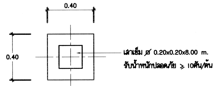
แปลนฐานราก F2
