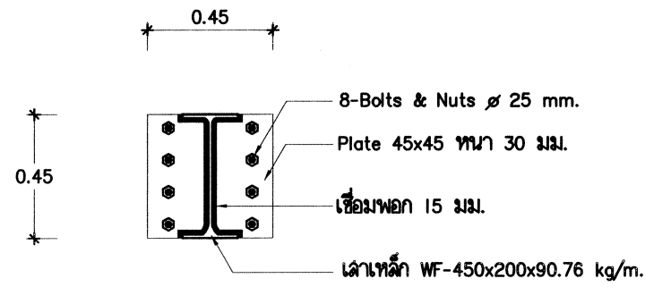
ขยายเล้า C-1
