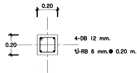
ขยายเล้า C2
