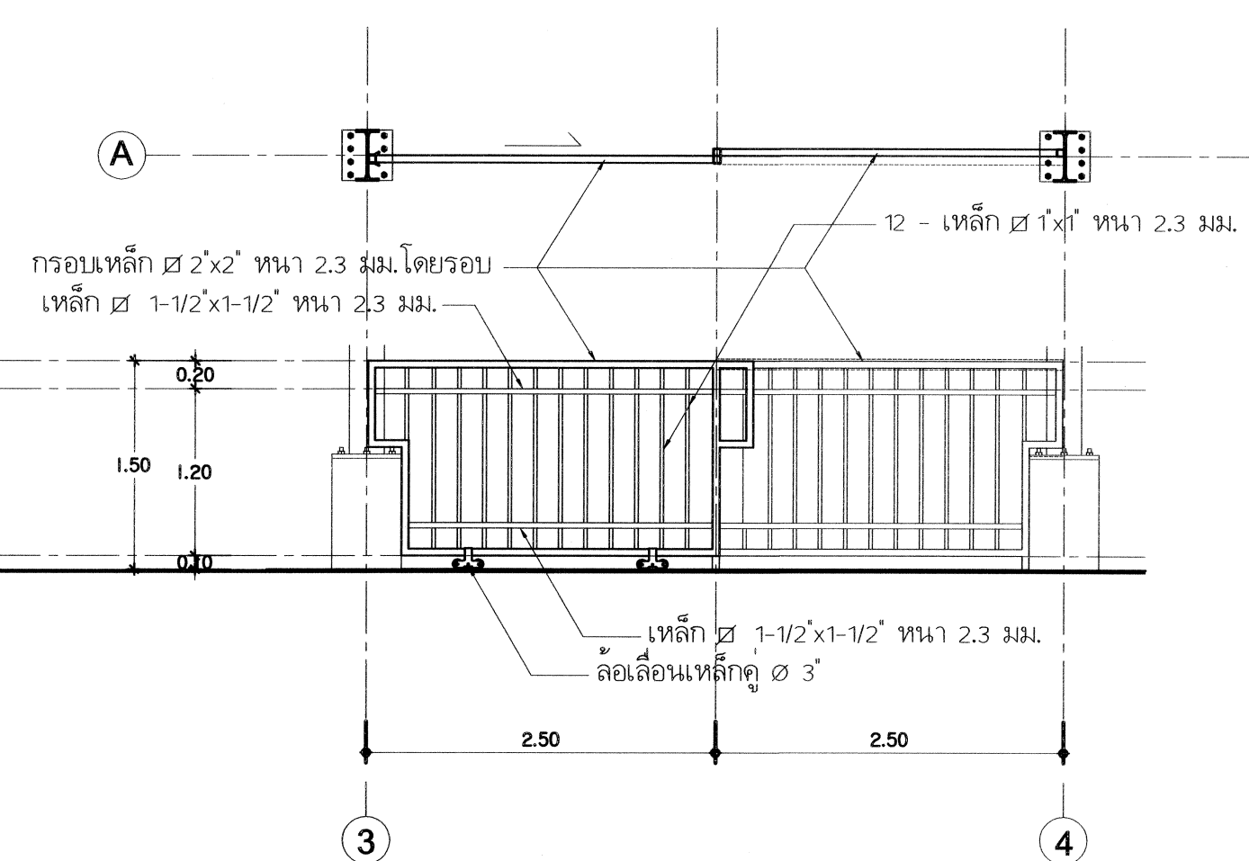
ขยายประตูบานเลื่อน ป มาตรฐาน 1:50
