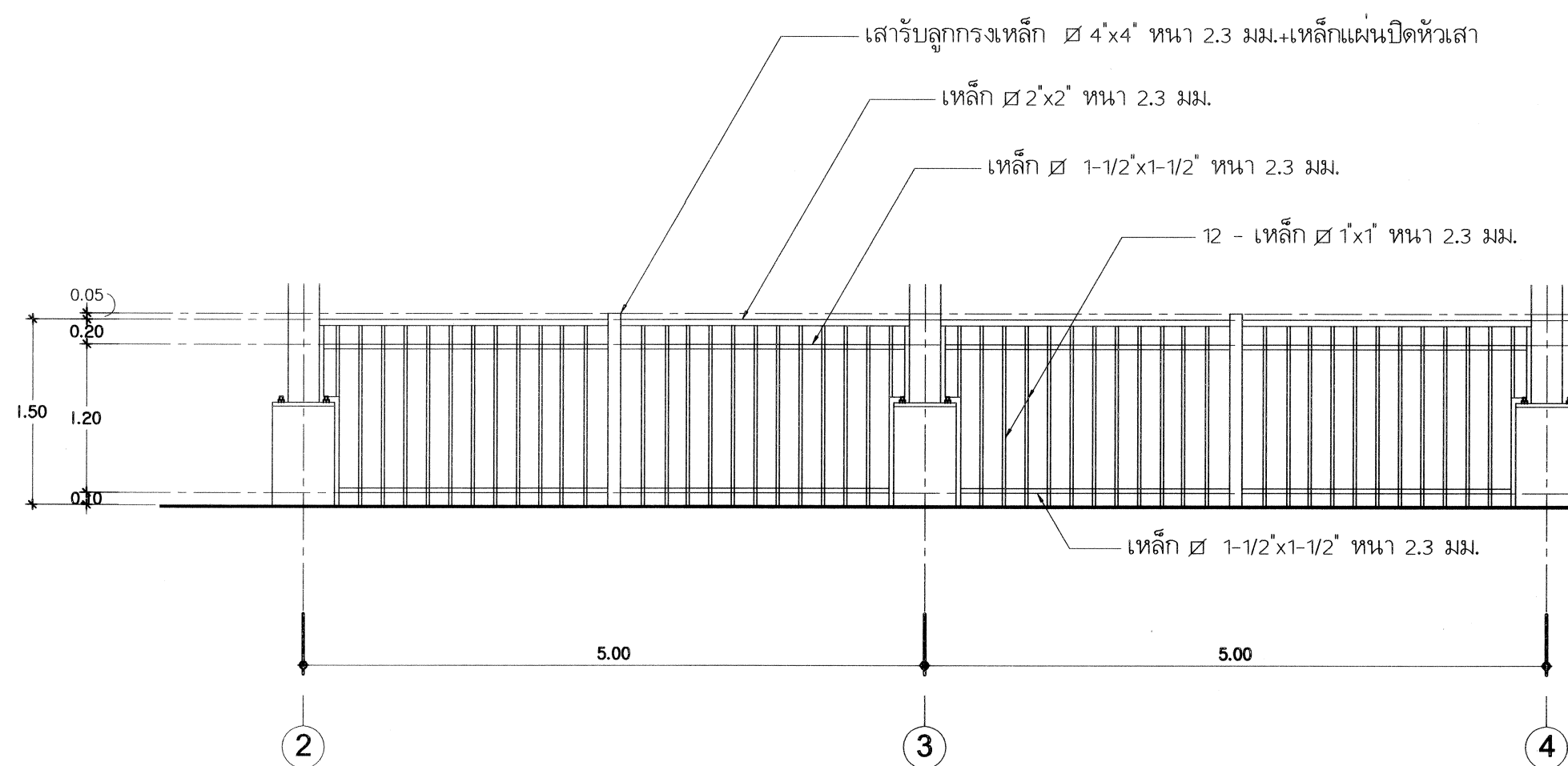
ขยายระบียงด้านยาว มาตรฐาน 1:50
