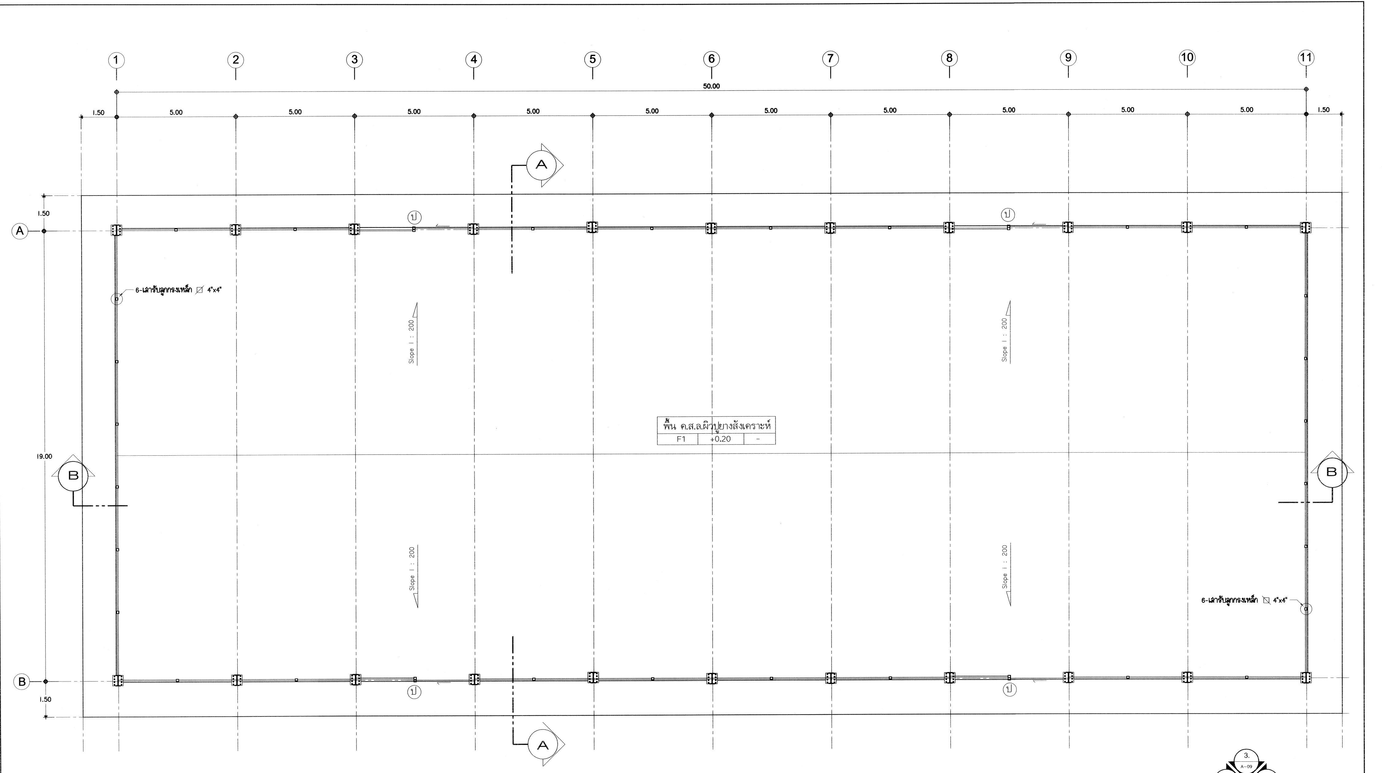
แปลนพื้น มาตราส่วน 1:100
