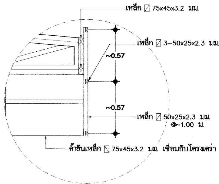
ขยาบโครงเคร่าเหล็กค้ำหลัง มาตราส่วน 1:25
