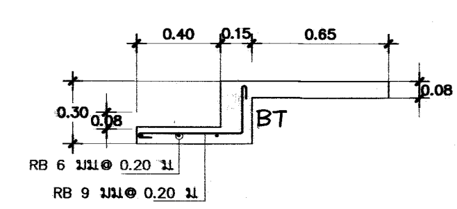
** คาน B หนาตัดเสมอเสาเอ็นล่างเหล็ก เข้าทั้งสองฝั่ง เสาเอ็นเสมอหลังคาน B ** รูปตัดขยายคานเคอร์ขยายอาหาร / 1:25
