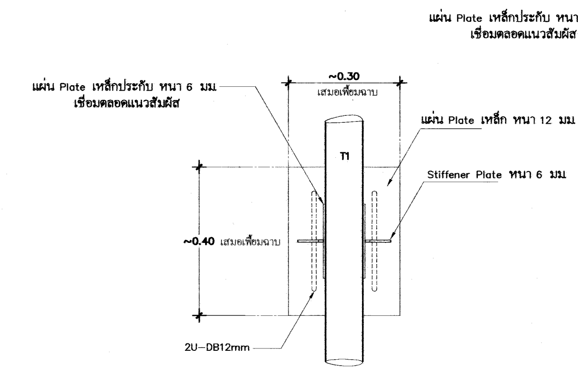
แปลนจตุรกรรับหัวเสา
