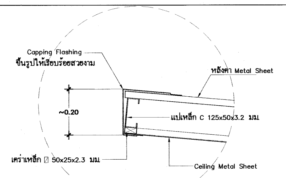
แบบขยายขยายคา 1 มาตราส่วน 1:10
