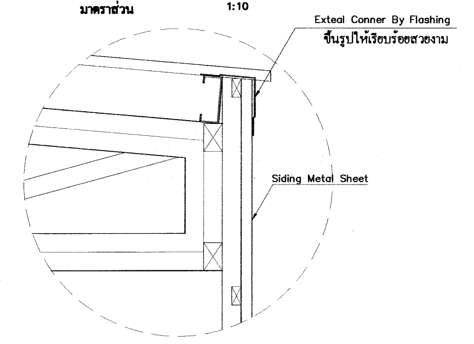
แบบขยายขยายคา 3 มาตราส่วน 1:10
