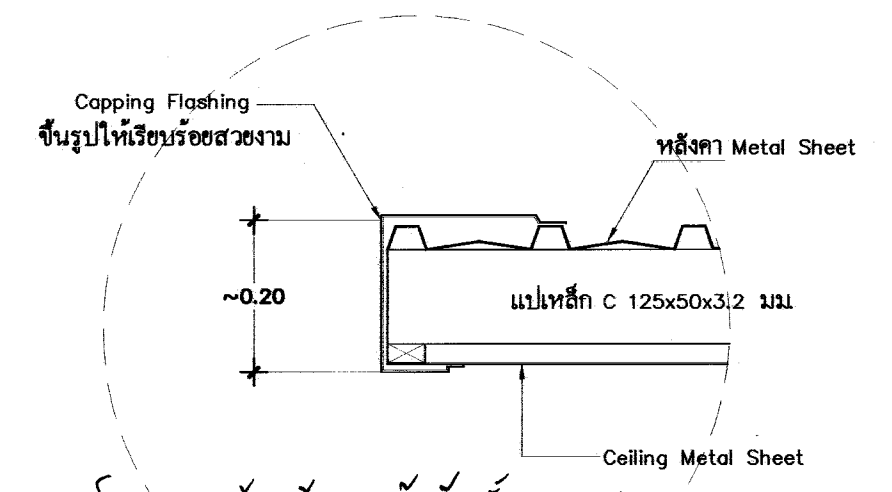
แบบขยายขยายคา 1 มาตราส่วน 1:10
