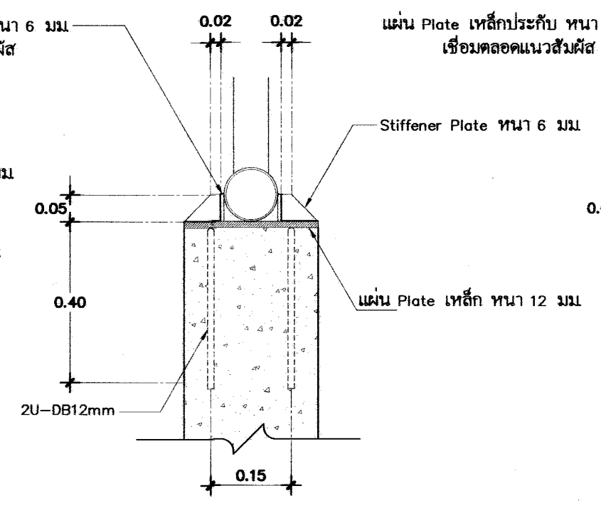
รูปตัด แสดงด้านหน้า
