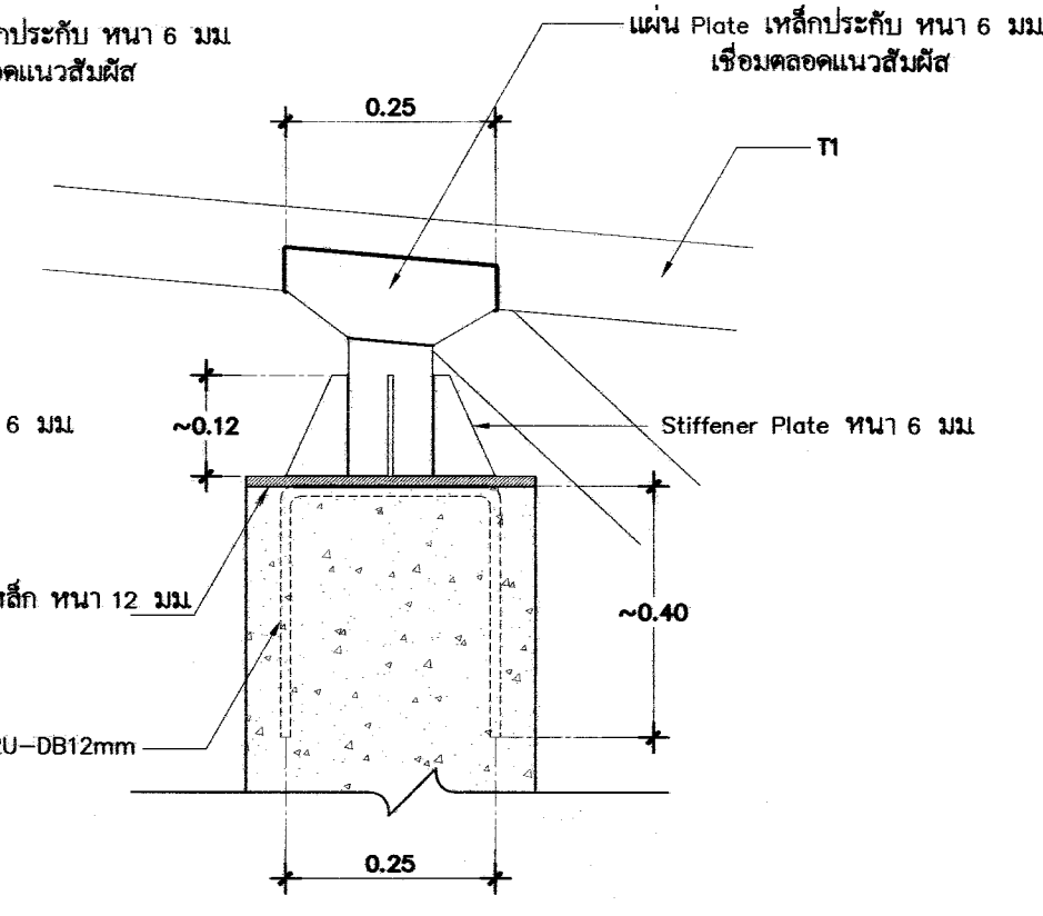
รูปตัด แสดงด้านข้าง
