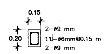
ขยายทับหลังประตู - หน้าค้ำ
