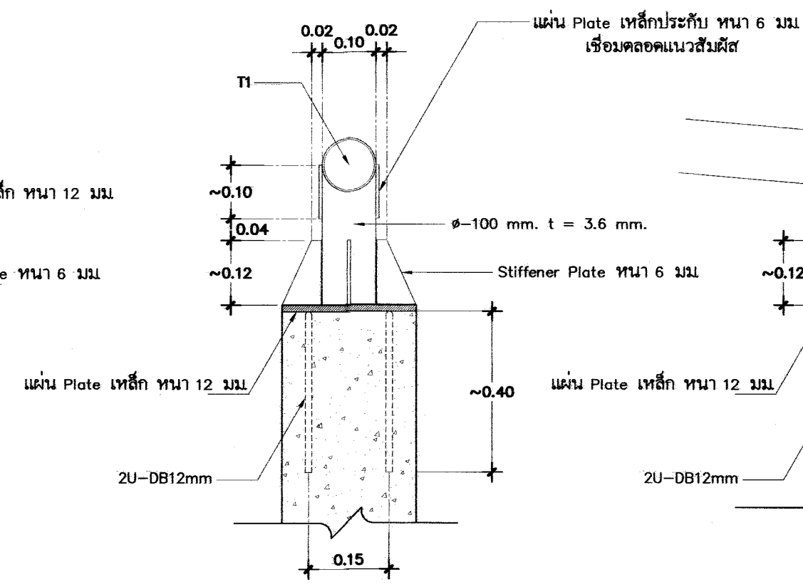
รูปตัด แสดงด้านหน้า
