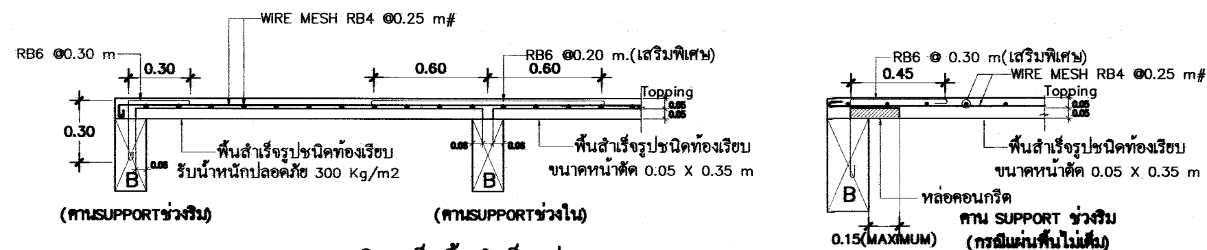
แบบขยายการเสริมเหล็กพื้นสำเร็จรูป
