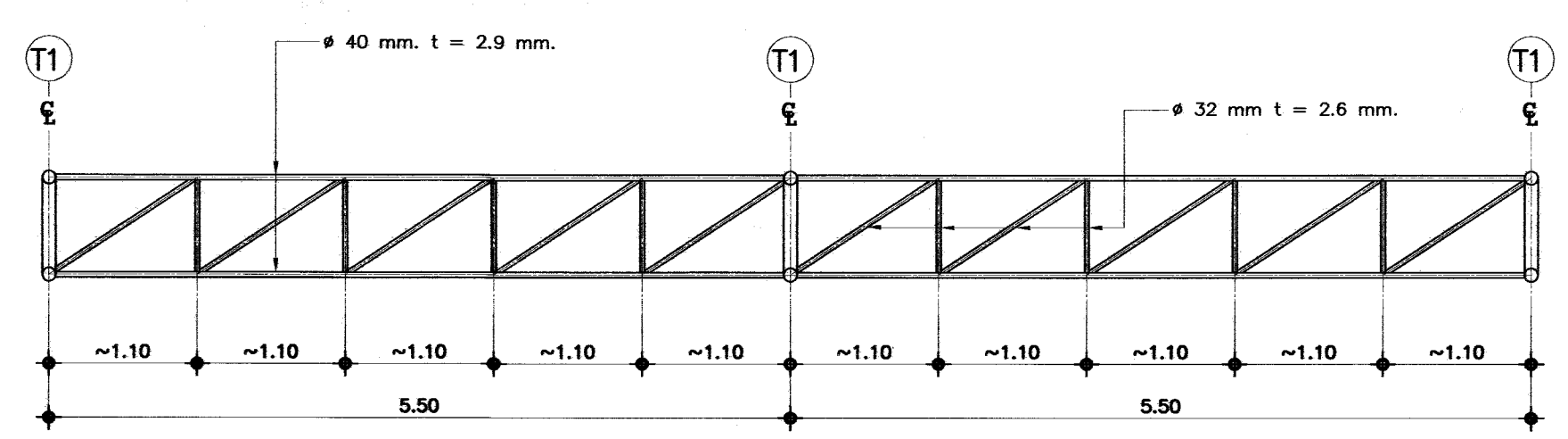
ขยาย T3 มาตราส่วน 1:50
