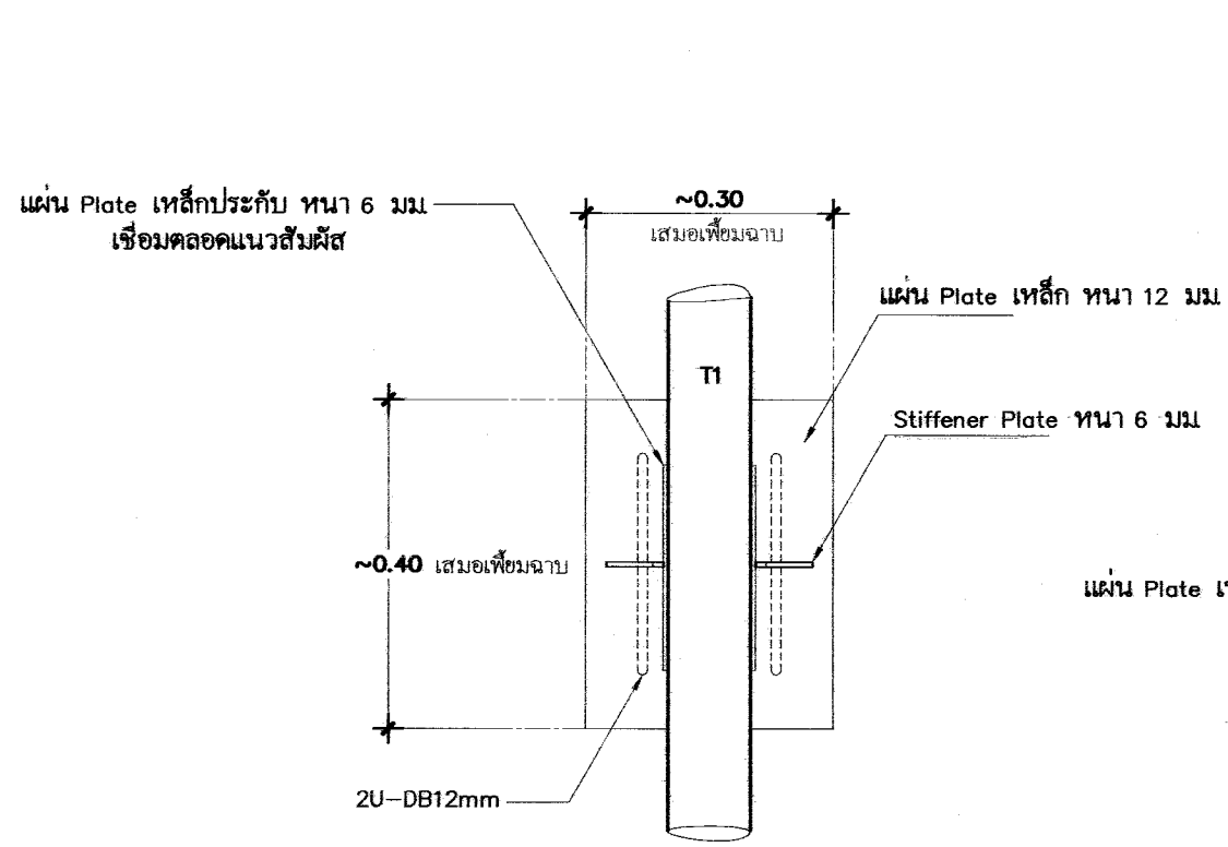
แปลนจตุรกรรับหัวเสา
