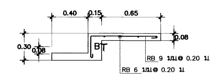
** คาน B หนาตัดเสมอเสาเอ็นล่างเหล็ก เข้าทั้งสองฝั่ง เสาเอ็นเสมอหลังคาน B ** รูปตัดขยายคานเคอร์ขยายอาหาร / 1:25
